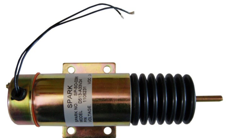
24V 2 FIS SYNCRO-START/TROMETTA SYNCRO-START PART NO: D513-A33V24
